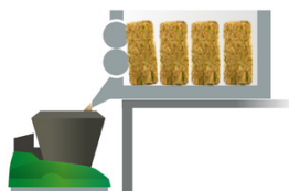
VARIANTA 2: PLNĚNÍ SHUTTLE ECO POMOCÍ PORTU (VOLNÝ PÁD NEBO DOPRAVNÍ PÁŠ)
